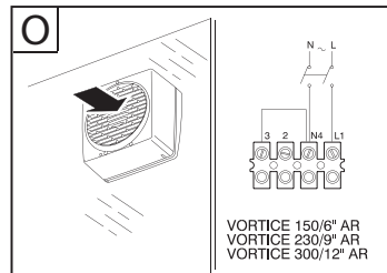
LUFT-EXTRAKTION AUS DEM SCHLAFZIMMER
