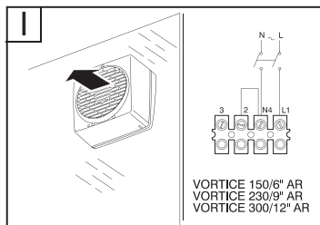
ENTRÉE D'AIR DE L'EXTÉRIEUR
